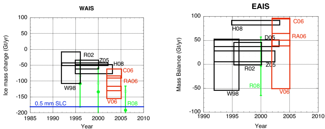
Figuur 1.7: Verschillende schattingen van de massabalans van de West Antarctische Ijskap (WAIS, links) en de Oost Antarctische Ijskap (EAIS, rechts). Bepaald uit groen – Insar metingen van de ijssnelheid; rood – zwaartekrachtmetingen (GRACE); zwart – radarhoogtemeting. De getallen corresponderen met het jaar van publicatie, de letter met de naam van de eerste auteur [W98 (Wingham et al., 1998), R02 (Rignot et al., 2002), D05 (Davis et al., 2005), Z05 (Zwally et al. 2005), C06 (Chen et al. 2006), RA06 (Ramilien et al. 2006), V06 (Velicogna et al. (2006), R08 (Rignot, 2008), H08 (Helsen et al., 2008)]
