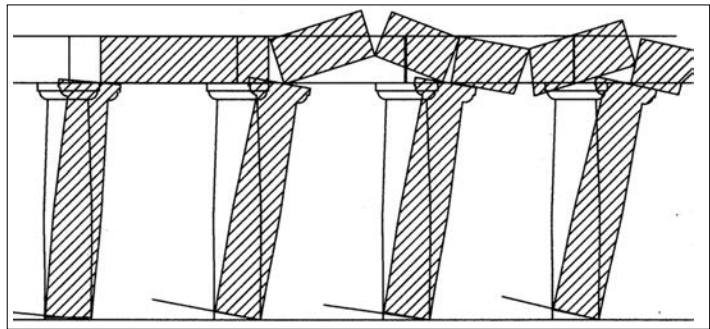
Fig. 3 – Selinunte, tempio C: l'effetto dell'urto sismico ortogonale alla peristasi del lato nord costituito da colonne di rocchi tozzi (prima dell'anastilosi).
