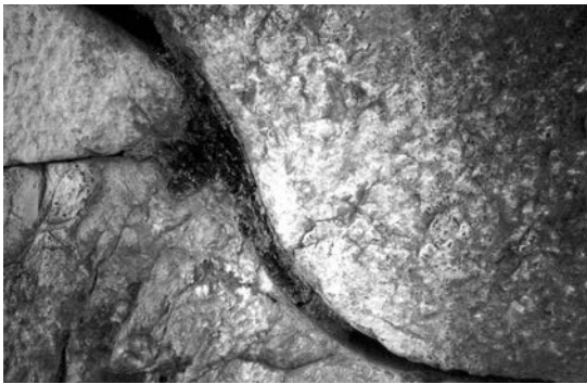
Fig. 46 – Delfi, sarcitura in piombo (con codolo anti slittamento) delle lesioni sismiche dell'opera poligonale nel santuario di Delfi.
