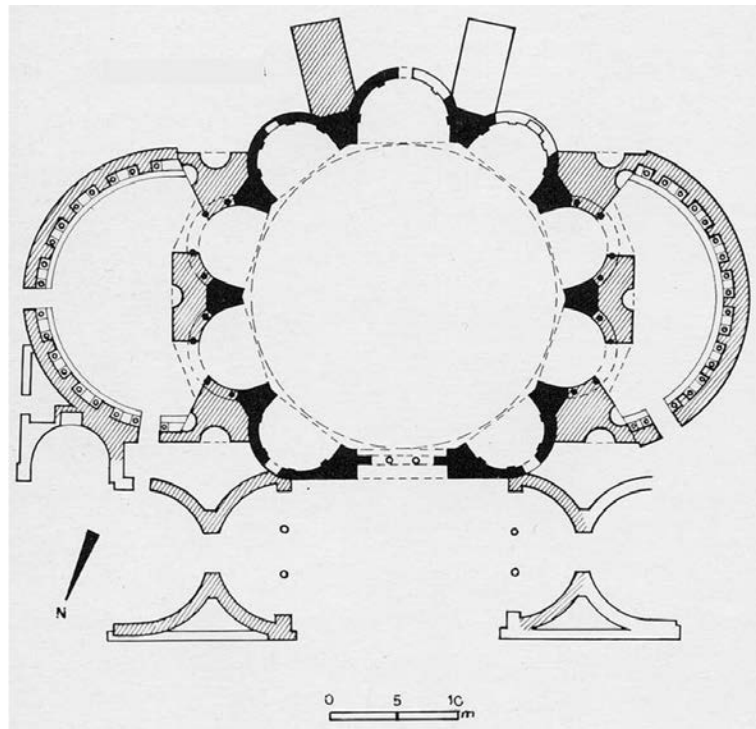
Fig. 15 – Roma, Minerva Medica, in nero pieno la struttura originaria.
