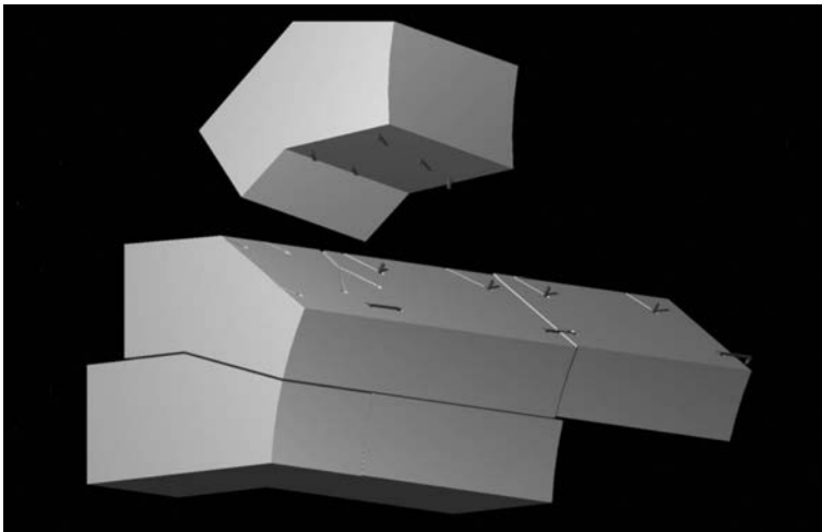
Fig. 42 – Roma, Ponte Cestio, il sistema di legamento dei blocchi.
