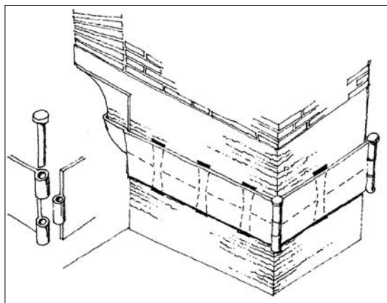
Fig. 69 – Proposta di ricostruzione del sistema per il fissaggio delle grappe attraverso una fascia metallica (bronzo) sagomata ad avvolgere anche la parte inferiore della mensola.
