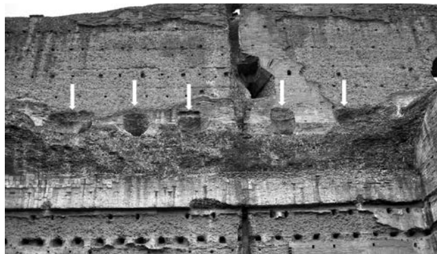
Fig. 54 – Roma, Terme di Caracalla, ricollocazione virtuale delle catene (C.M.Amici).
