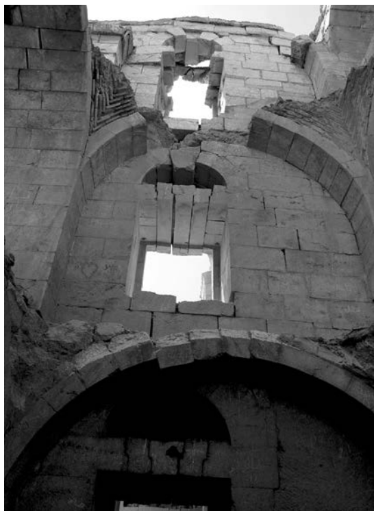
Fig. 7 – Siria, Halabye: pretorio; è evidente la maggiore entità delle lesioni con l'aumentare dell'altezza dovute all'effetto "pendolo rovescio".
