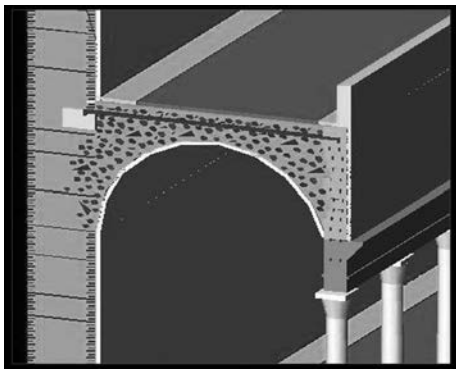
Fig. 54 – Roma, Terme di Caracalla, ricollocazione virtuale delle catene (C.M.Amici).
