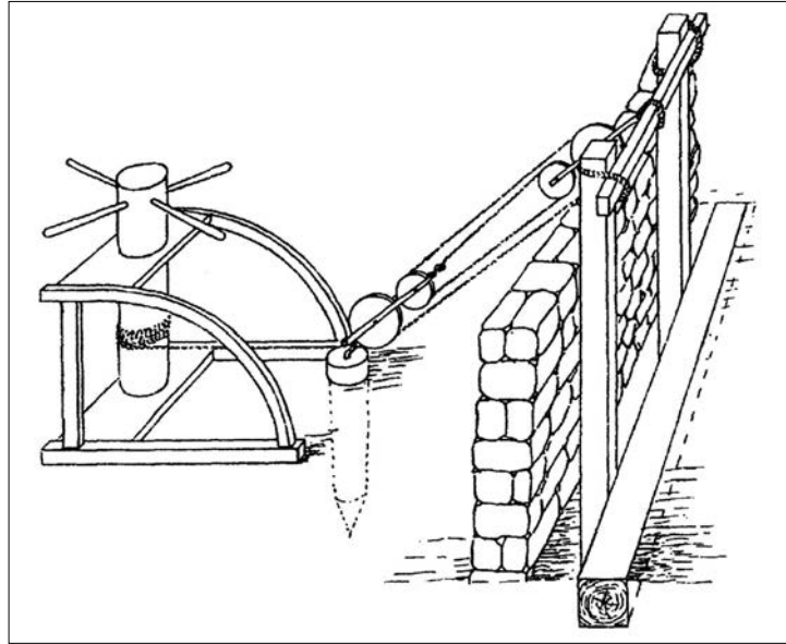
Fig. 11 – Sistema per raddrizzare una parete strapiombata (da Erone di Alessandria).
