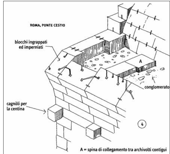
Fig. 42 – Roma, Ponte Cestio, il sistema di legamento dei blocchi.
