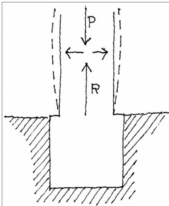
Fig. 2 – Tendenza a spanciamento per risultante di trazione.
