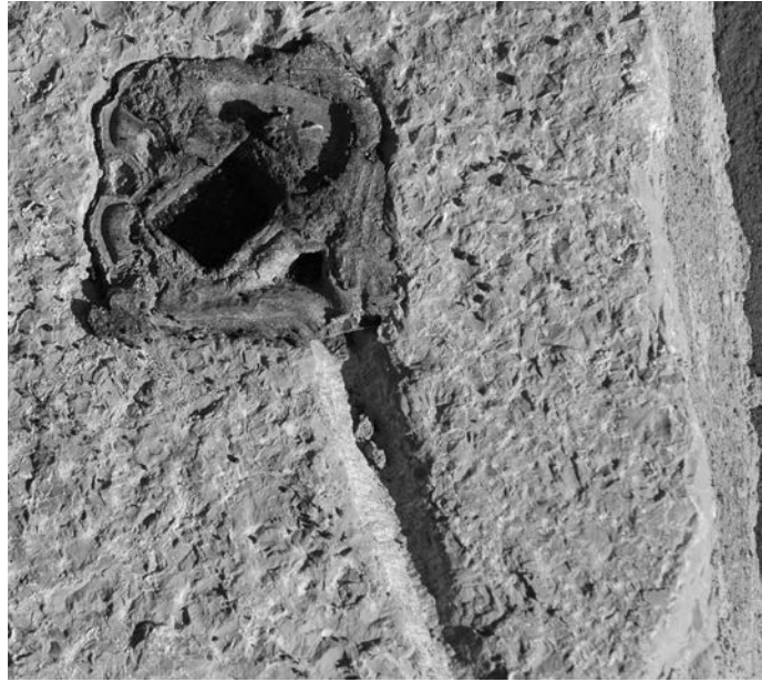
Fig. 48 – Piombatura di perno sulla faccia d'attesa di un blocco.
