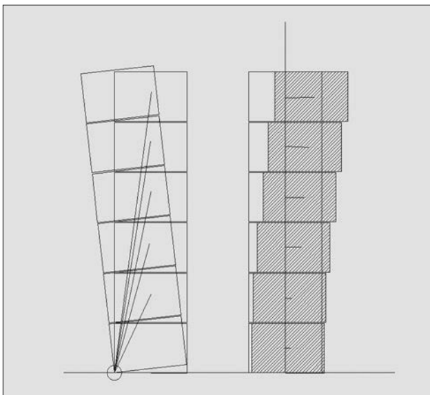
Fig. 5 – Cinematismo della colonna a rocchi tozzi, a destra, posizione a seguito dell'urto.
