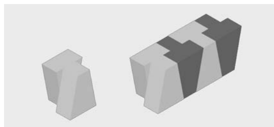
Fig. 36 – Conci di piattabande nell'architettura islamica. Fig. 37 – Concio singolo e assemblaggio dei blocchi della piattabanda del Duomo di Prato.
