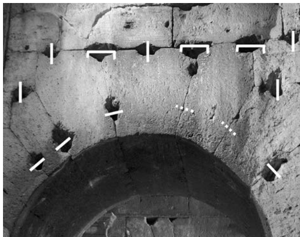
Fig. 43 – Modello dei conci di un arco con grappe e perni.
