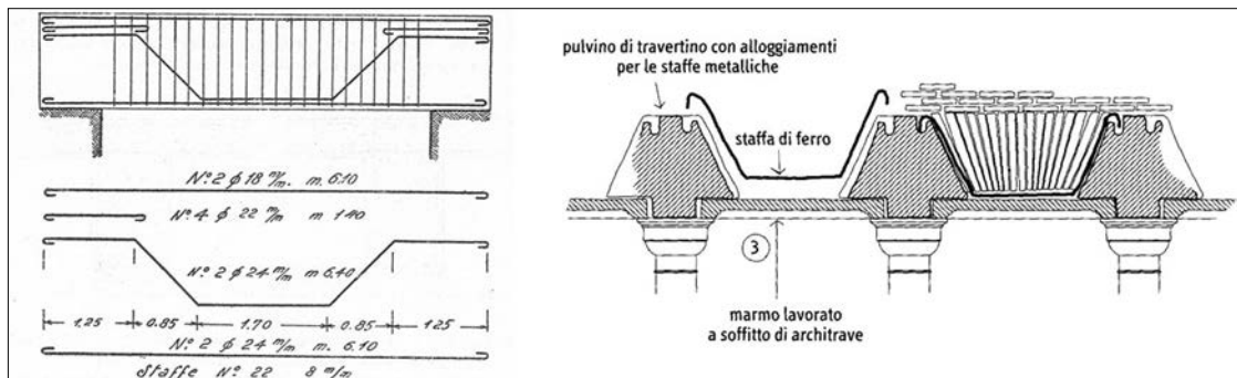
Fig. 59 – Schema dei ferri in un architrave in conglomerato armato e nella piattabanda armata antica.
