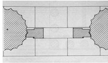
Fig. 61 – Selinunte, tempio F, parziale chiusura degli intercolumnni con parete di seconda fase piena e finestrata.
