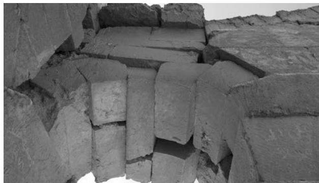
Fig. 40 – Siria, Halabye, pretorio di età bizantina, dislocazione dei blocchi per effetto del sisma.
