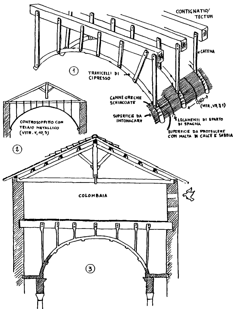
FIGURA 3.12 Controsoffittature
