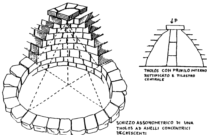
FIGURA 3.4 Pseudo cupola
