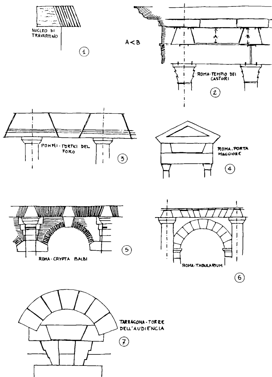
FIGURA 3.23 Piattabanda
