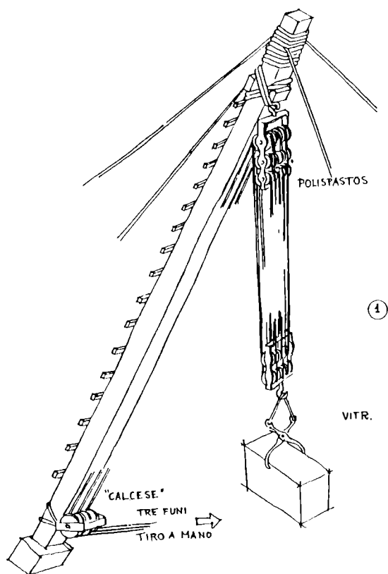
FIGURA 8.5 Macchine elevatorie
